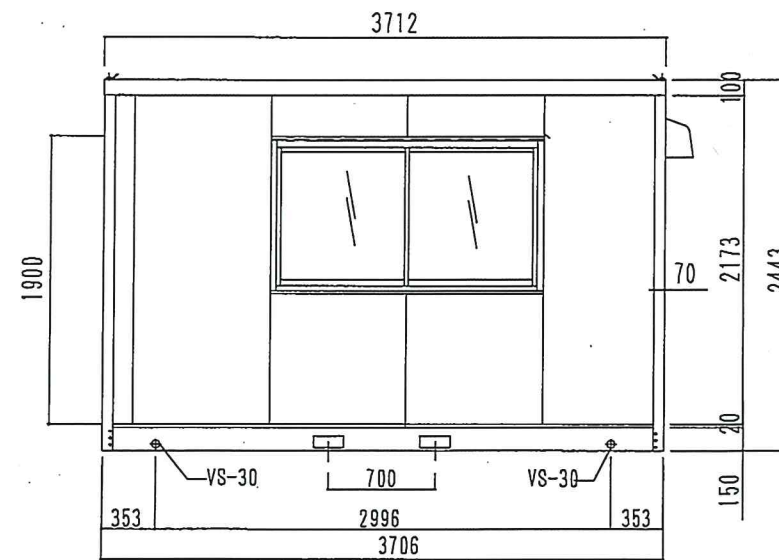
背面図
