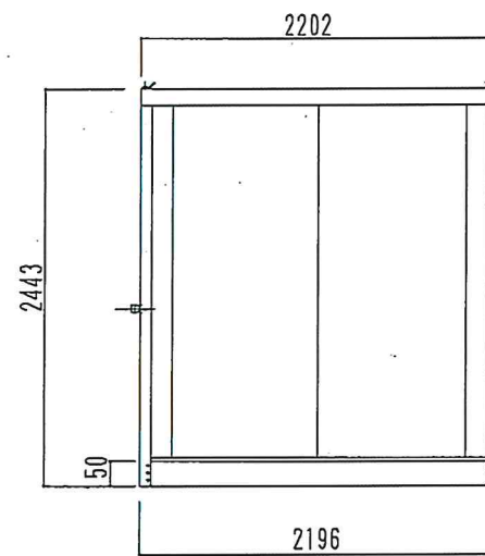
右側面図
