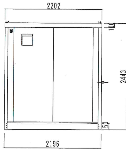
左側面図
