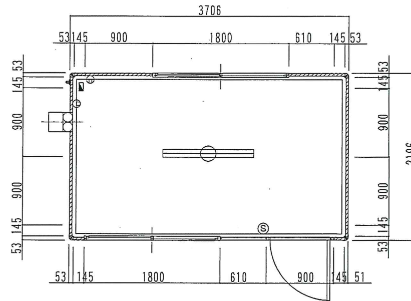
平面図
