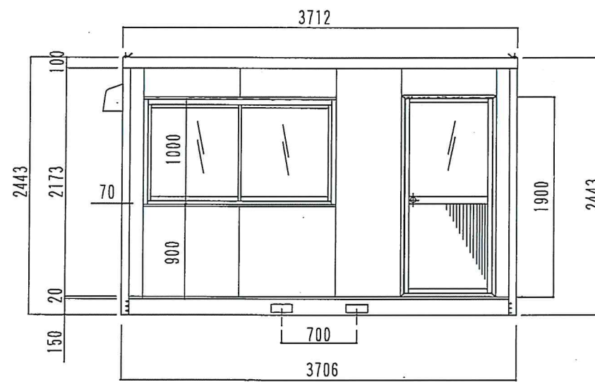
正面図
