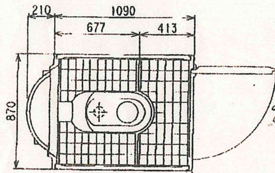
平面図 (S=1/20)
