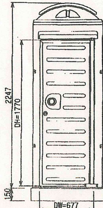
正面図 (S=1/20)
