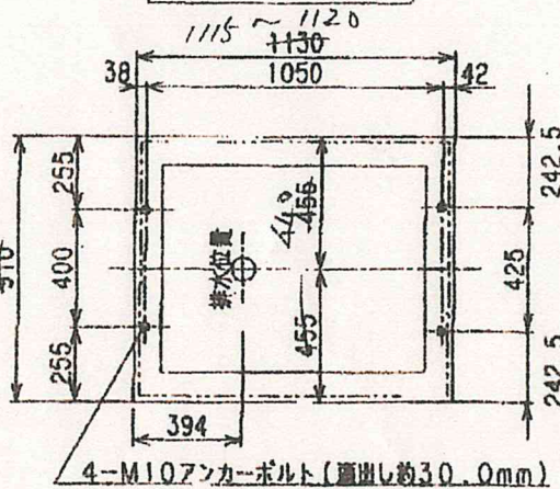
基礎図 (S=1/20)
