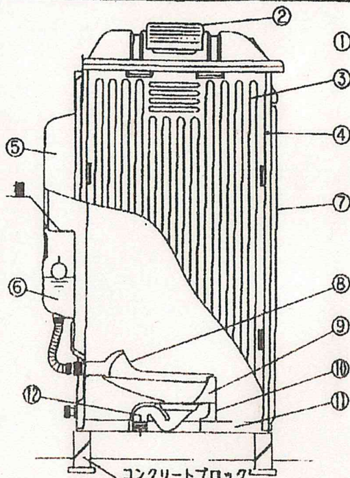
断面図 (S=1/20)
