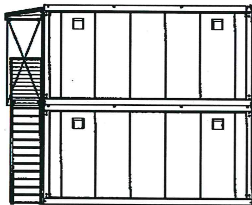
側面図
