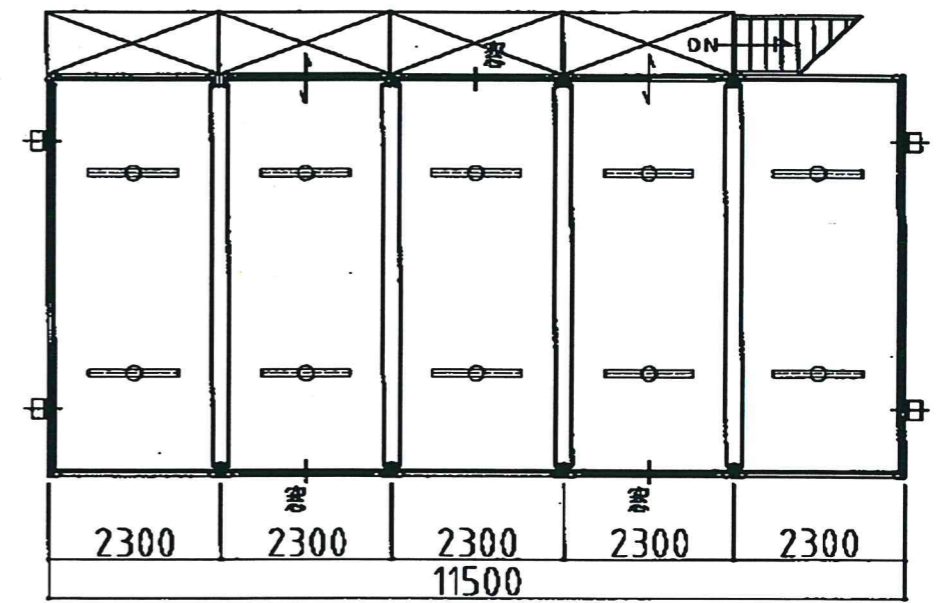
2F 平面図
