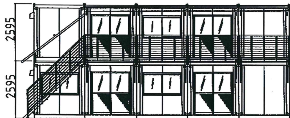
背面図
