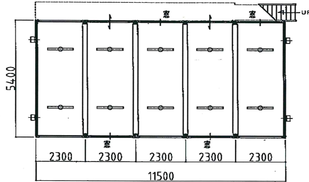
1F 平面図
