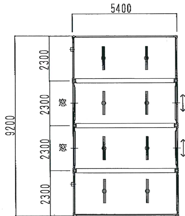
平面図
