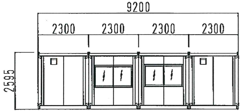
側面図
