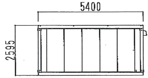
背面図
