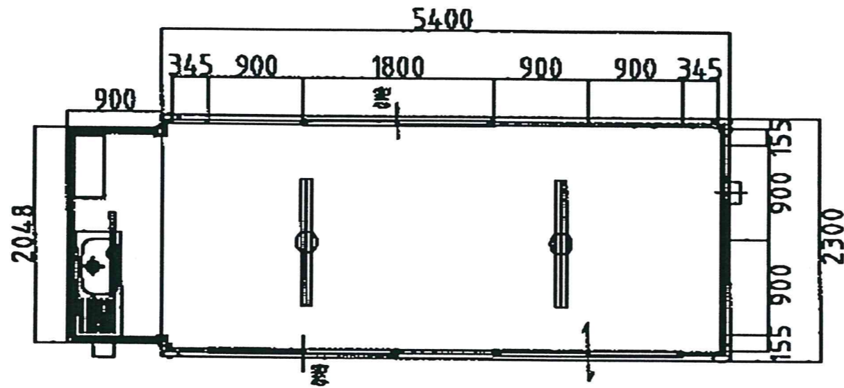
平面図
