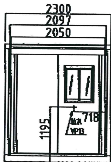
左側面図
