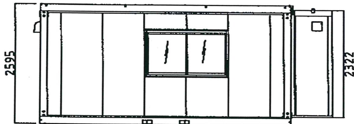
背面図
