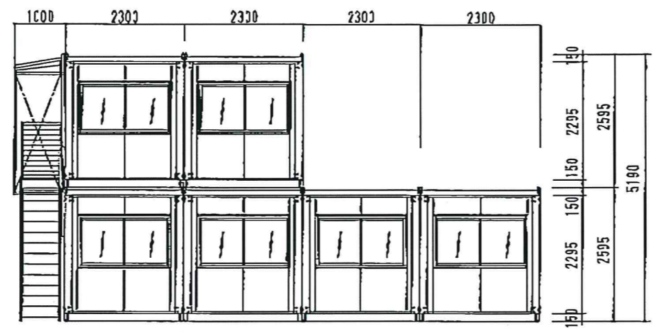
背面図
