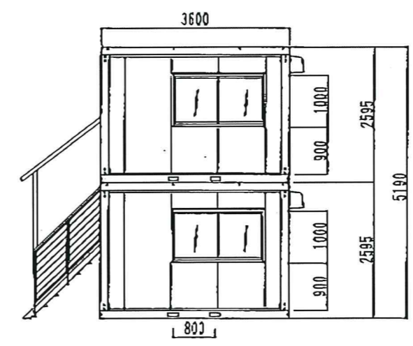
左側面図
